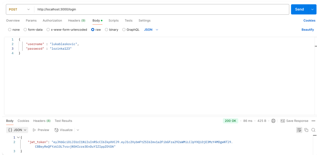
Slika 20. (Korak 4: Uspješna prijava korisnika, šaljem JWT token kao odgovor)
